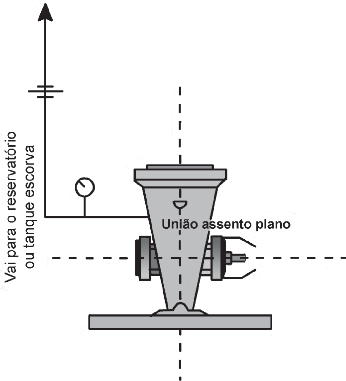
Figura C.7: Arrefecimento da bomba principal elétrica
