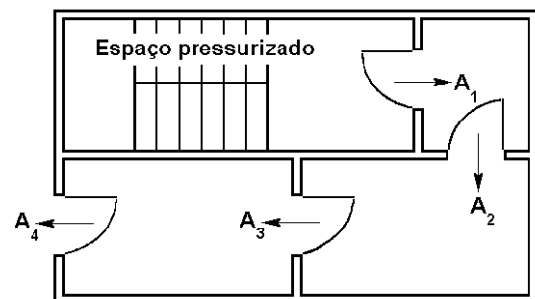
Figura 2: Trajetórias de escape do ar em série
