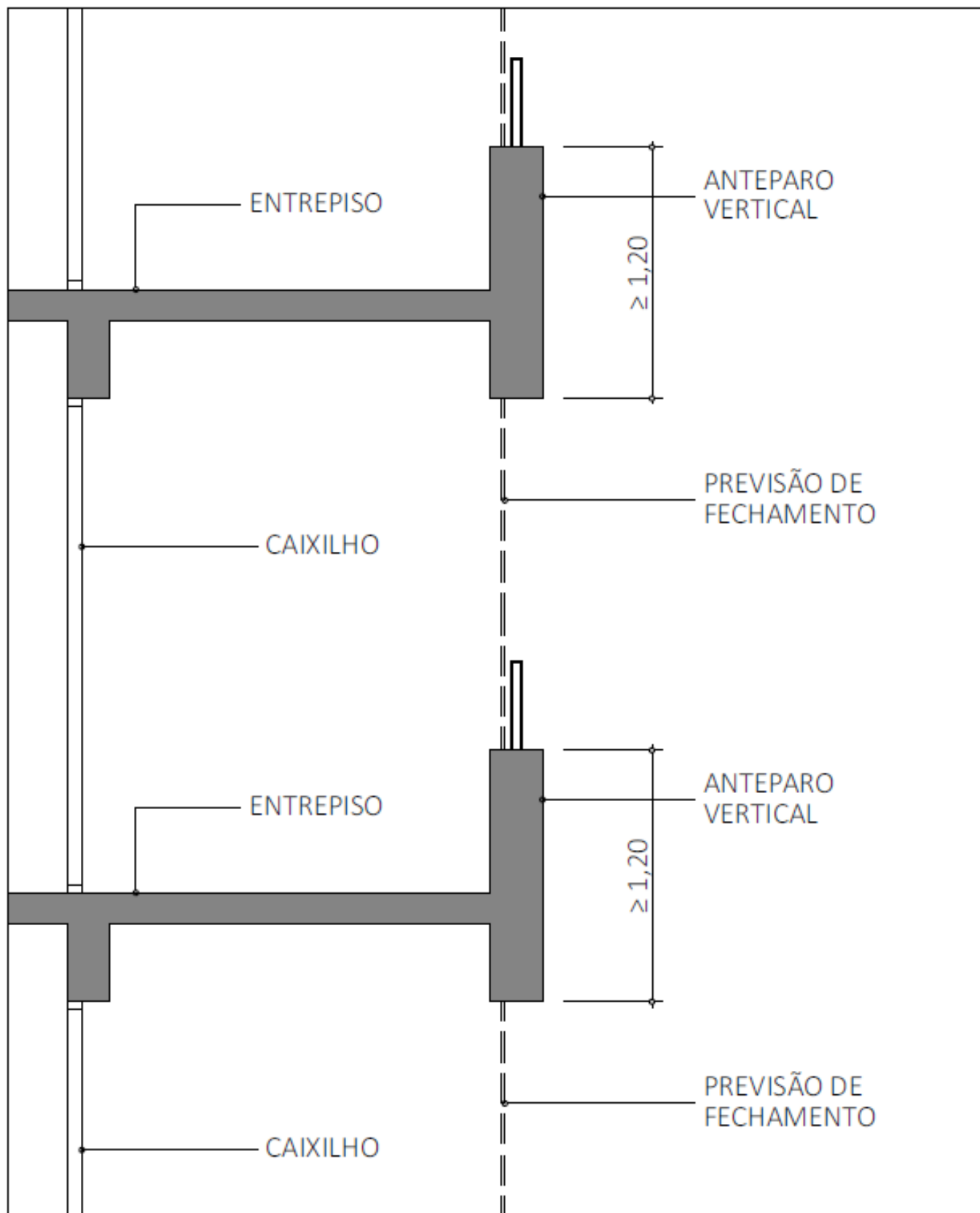
Figura A6: Modelo de fechamento com vidro
