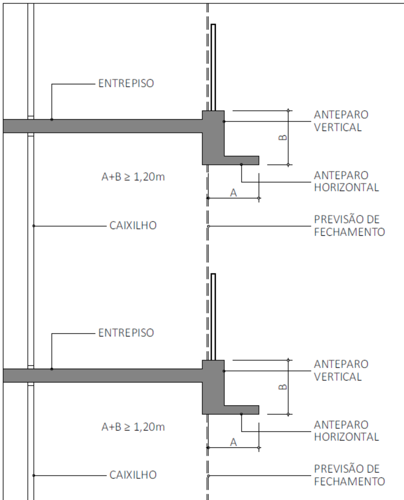
Figura A8: Modelo de fechamento com vidro
