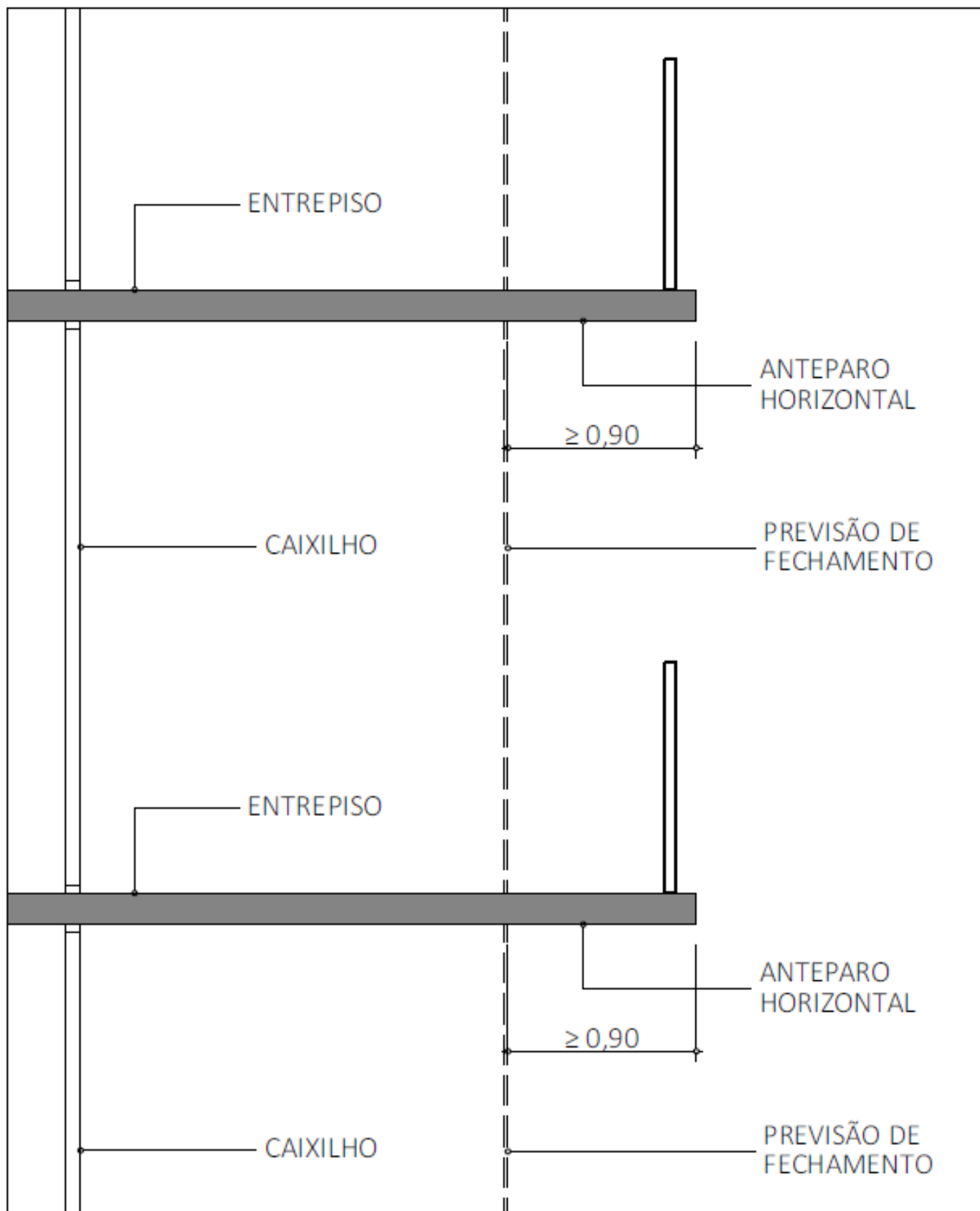
Figura A7: Modelo de fechamento com vidro
