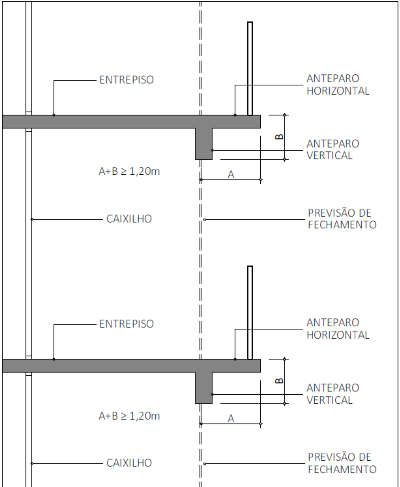
Figura A9: Modelo de fechamento com vidro
