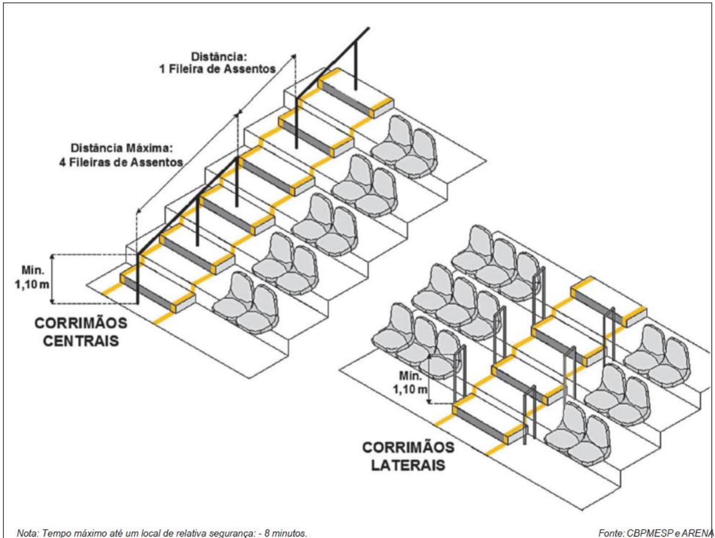
Figura 12: Perspectiva de corrimãos centrais e laterais
