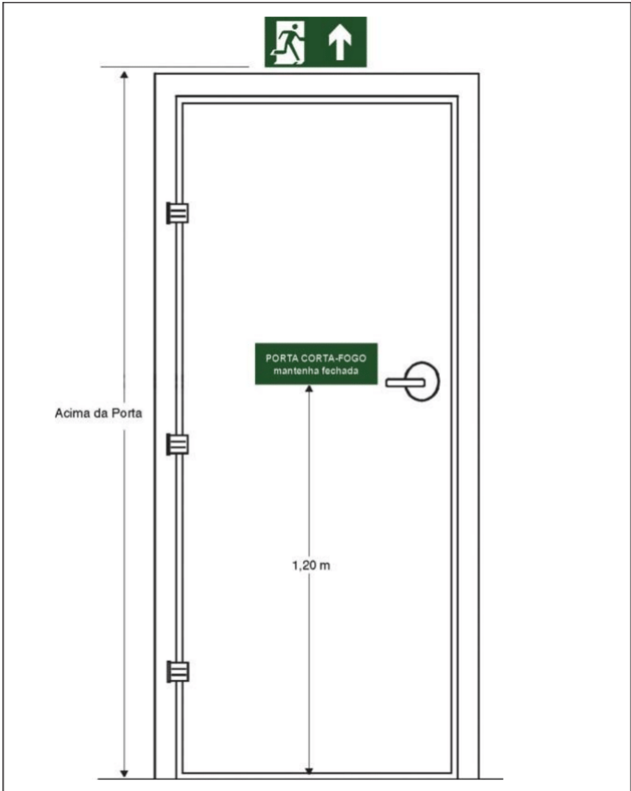
Figura C-1: Sinalização de porta corta-fogo (vista do hall )
