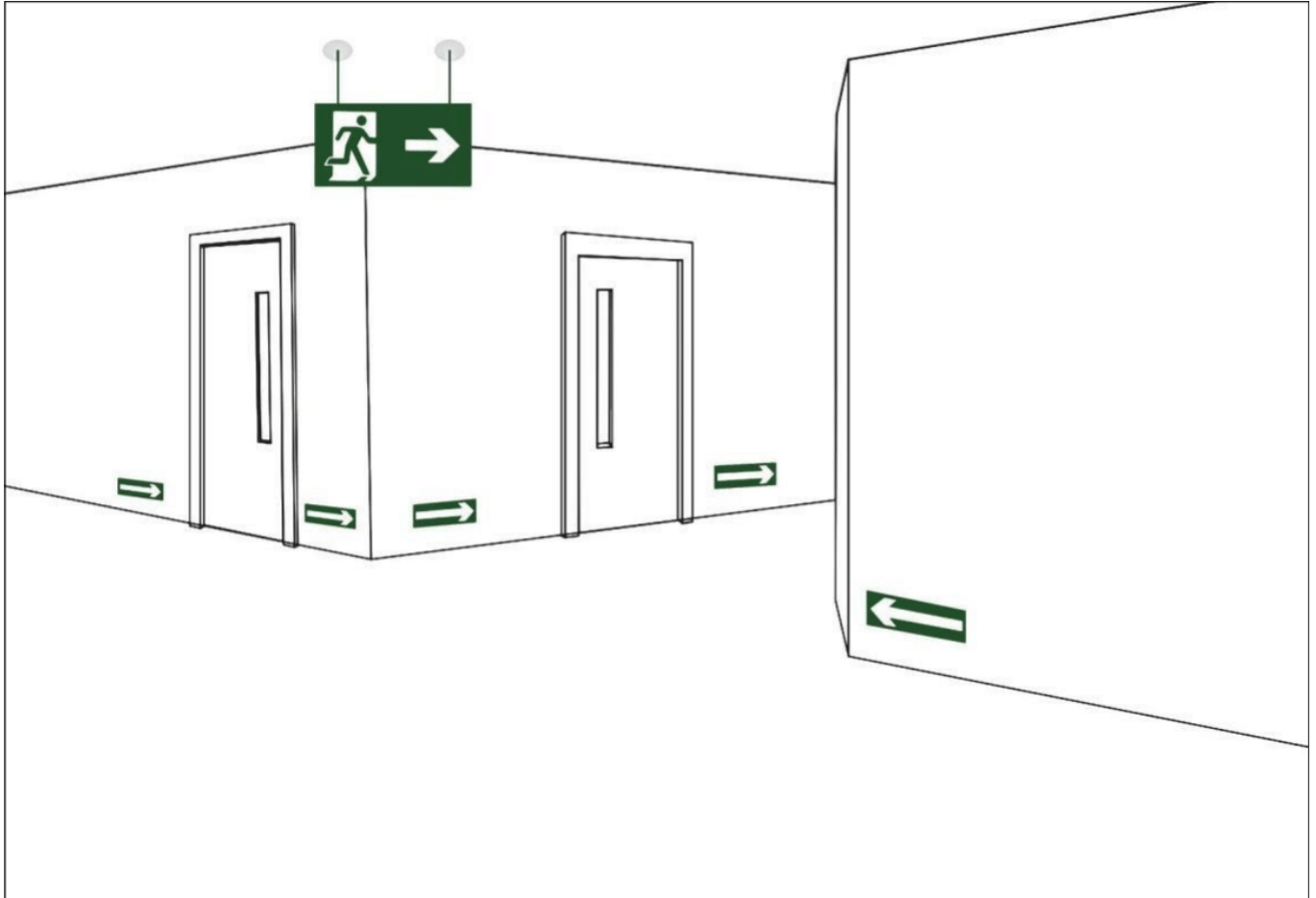
Figura C-13: Sinalização de saída perpendicular ao sentido da fuga, em dupla face
