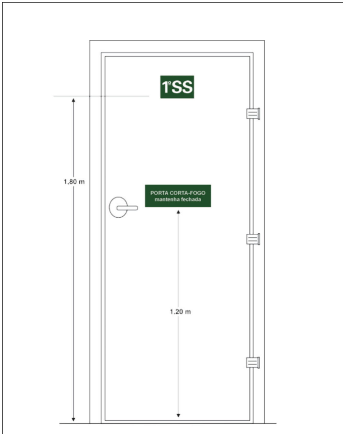
Figura C-2: Sinalização de porta corta-fogo (vista da escada)
