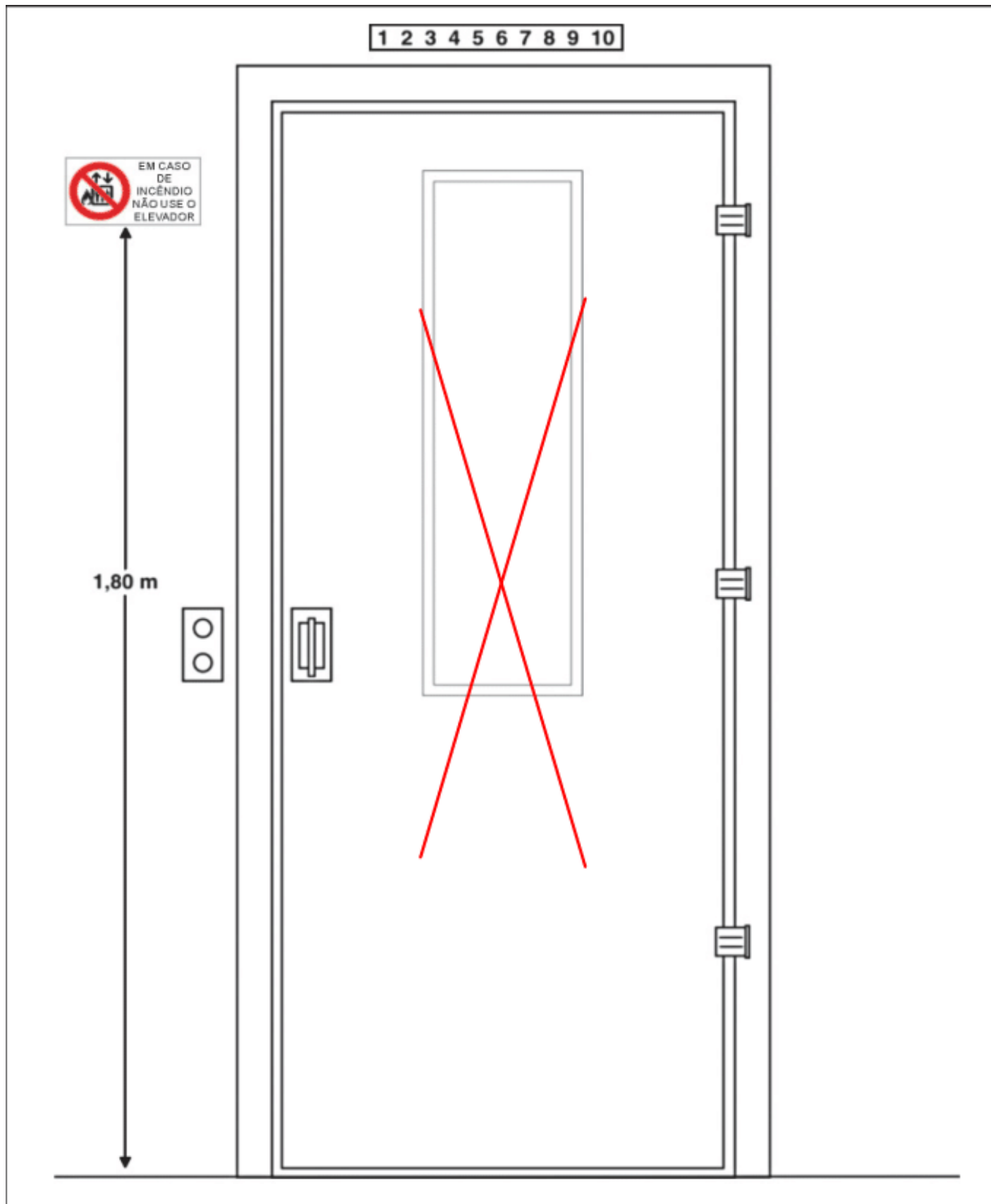
Figura C-4: Sinalização de elevadores (vista do hall )
