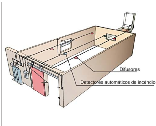
Figura 73: Sistema de CO 2
