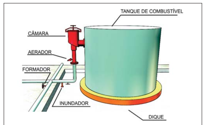
Figura 72: Detalhe de câmara de espuma
