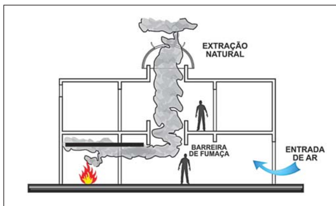
Figura 28: Extração de fumaça de átrios
