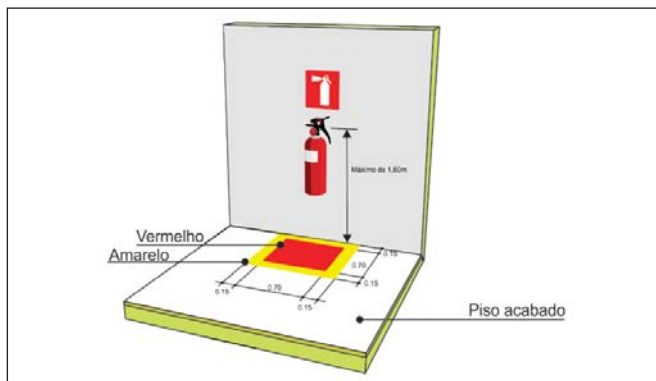
Figura 62: Detalhe de instalação de extintores em áreas sujeitas a obstrução
