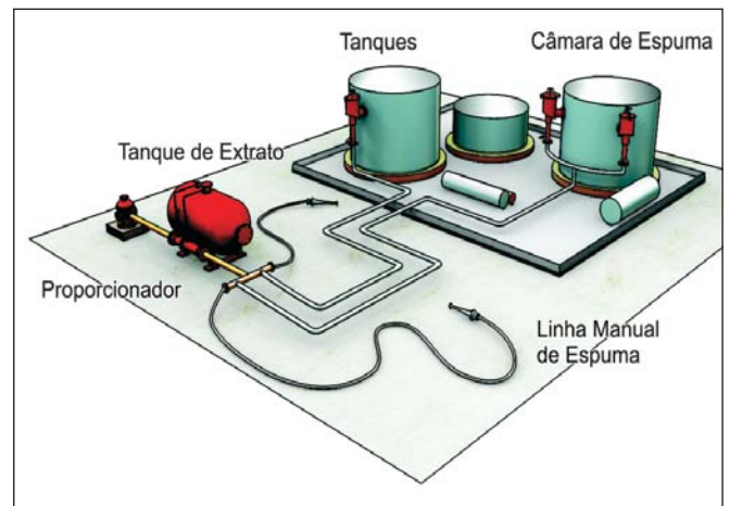
Figura 71: Sistema semifixo
