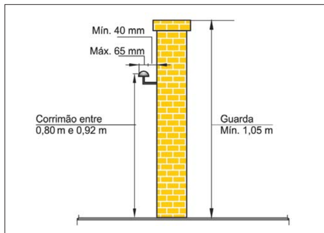
Figura 14: Dimensões de guardas e corrimãos
