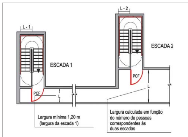
Figura 19: Dimensionamento de corredores de descarga
