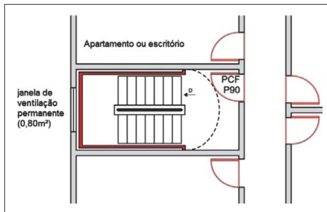
Figura 7: Escada enclausurada protegida
