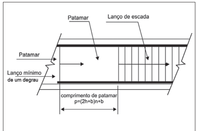
Figura 6: Lanço mínimo e comprimento de patamar
