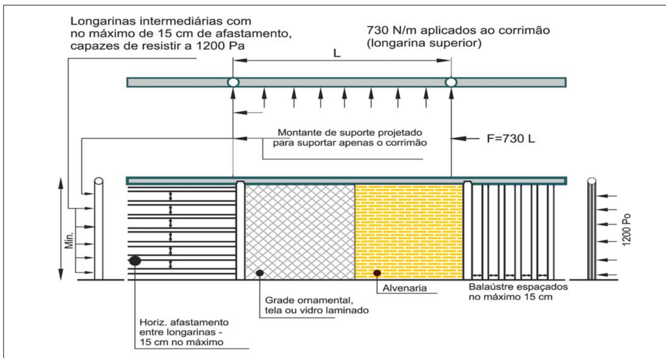
Figura 16: Pormenores construtivos da instalação de guardas e as cargas a que elas devem resistir
