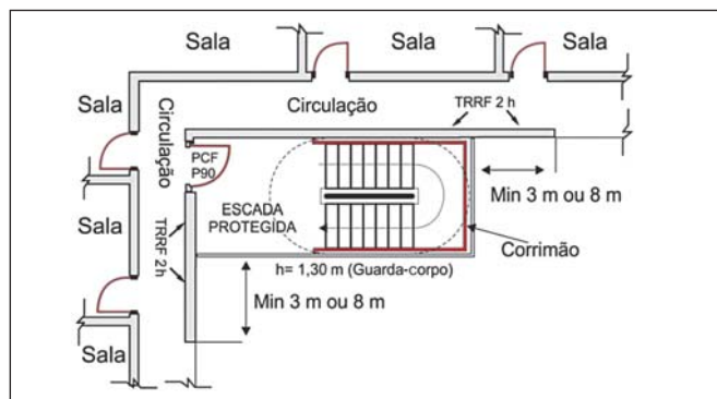
Figura 13: Escada aberta externa
