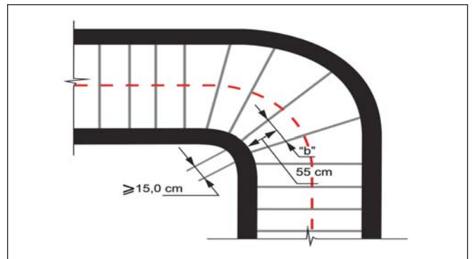
Figura 5: Escada com lanços curvos e degraus balanceados
