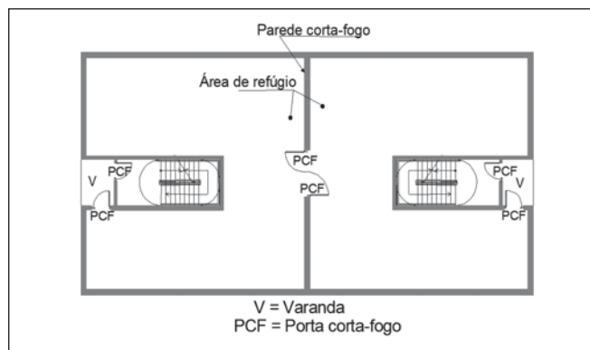
Figura 17: Desenho esquemático da área de refúgio
