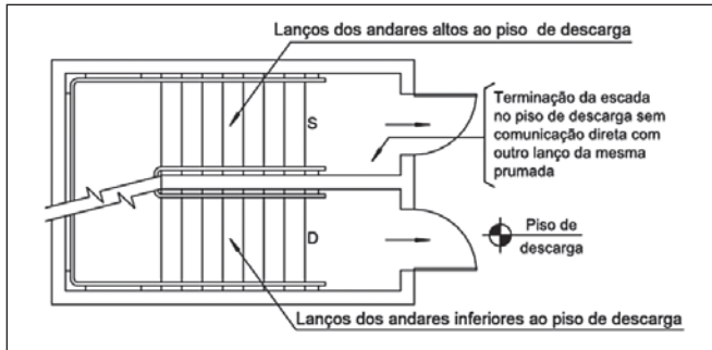
Figura 3: Segmentação das escadas no piso da descarga
