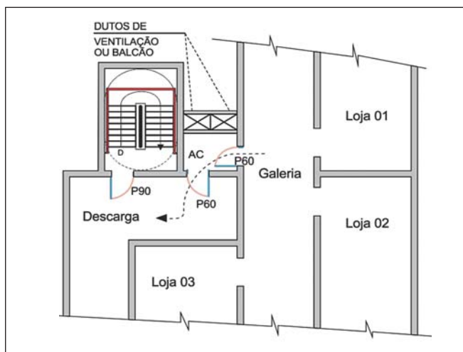
Figura 20: Acesso de galeria comercial à descarga
