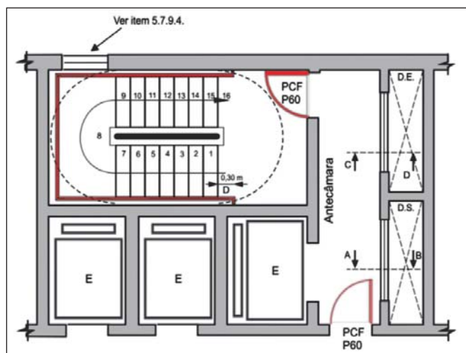
Figura 9: Escada enclausurada à prova de fumaça
