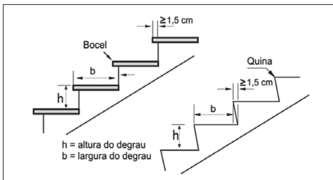
Figura 4: Altura e largura dos degraus
