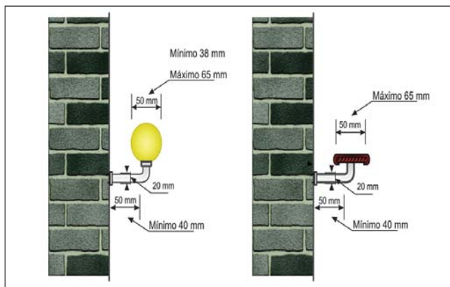
Figura 15: Pormenores de corrimãos
