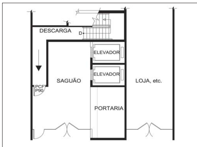
Figura 18: Descarga através de hall térreo não enclausurado
