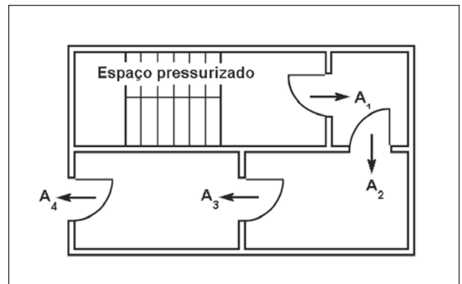
Figura 2: Trajetórias de escape do ar em série
