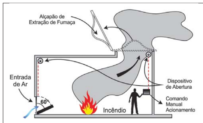
Figura 10: Ângulo de abertura dos obturadores
