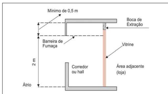
Figura 8: Detalhe de barreira de fumaça - corte
