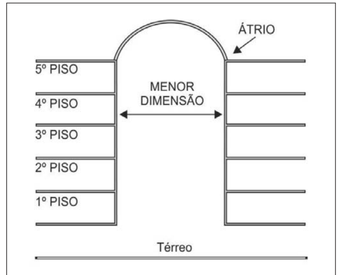
Figura 29: Modelo 1 de átrios cobertos fechados
