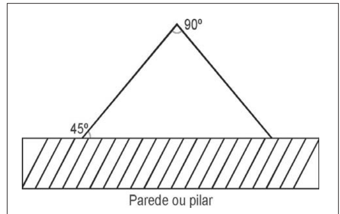
Figura 1: Instalação de placa angular
