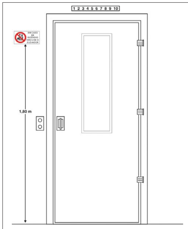
Figura C-4: Sinalização de elevadores (vista da escada)
