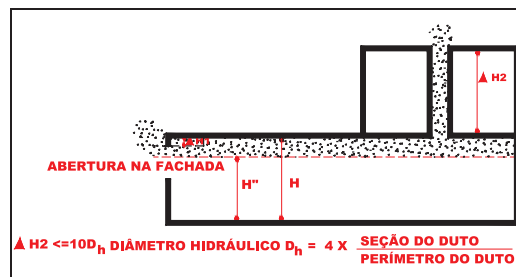
Figura 17 - Diâmetro hidráulico
