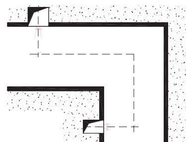
Figura 26 - Distância de extração de aberturas em trajeto diverso
