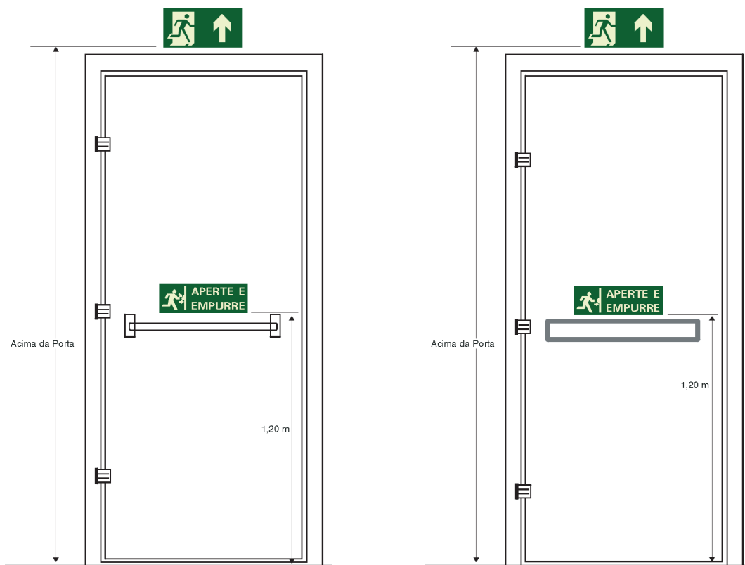
Figura 5 - Sinalização de portas com barras antipânico (modelos 1 e 2)
