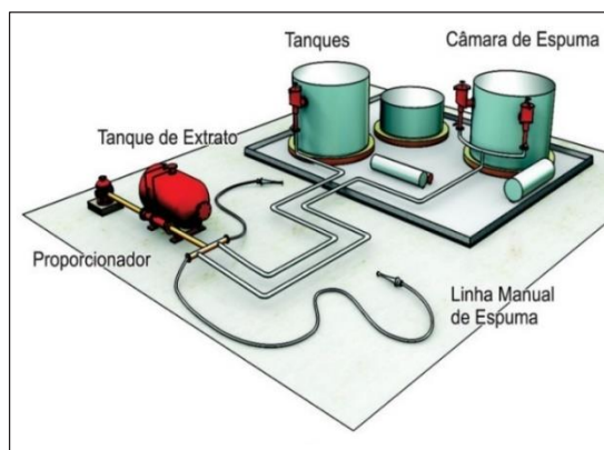
Figura 61: Sistema semifixo
