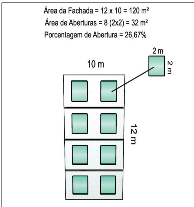
Figura 11: Porcentagem de aberturas na fachada
