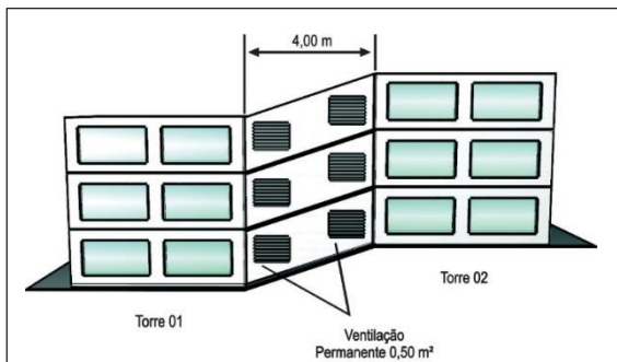
Figura 12: Abertura lateral na escada
