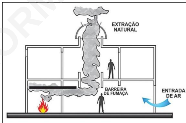
Figura 26: Extração de fumaça de átrios.
