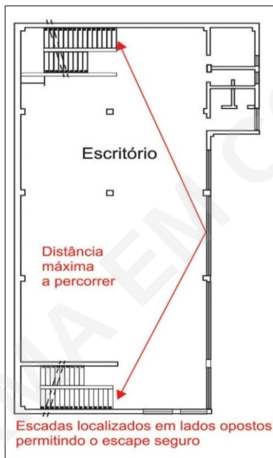
Figura 38: Localização e caminhamento para acesso a uma escada.
