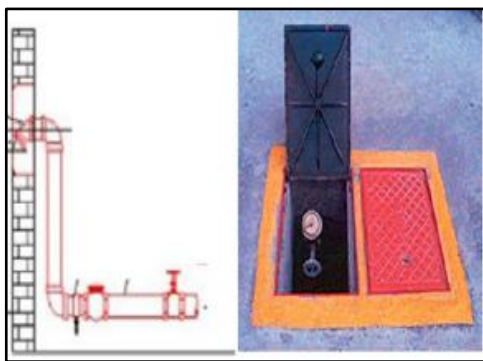
Figura 55: Registro de recalque de coluna e de passeio para bombeiros.
