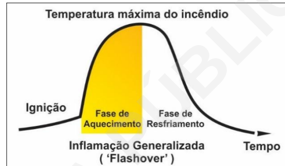
Figura 18: Curva temperatura-tempo de um incêndio.
