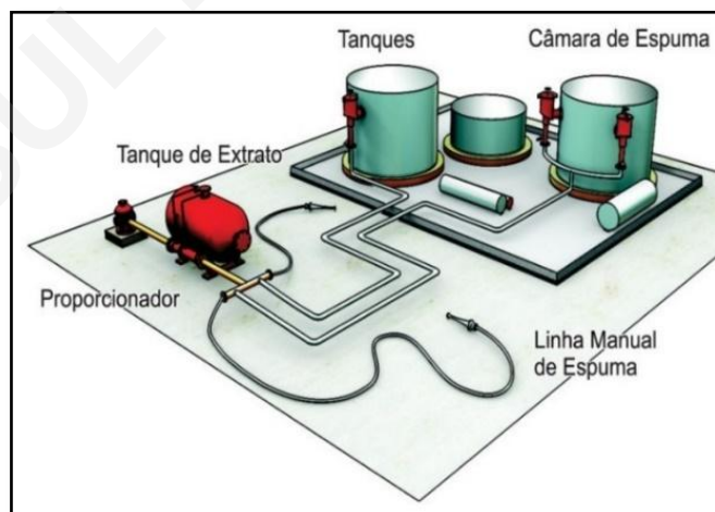
Figura 62: Sistema semifixo.
