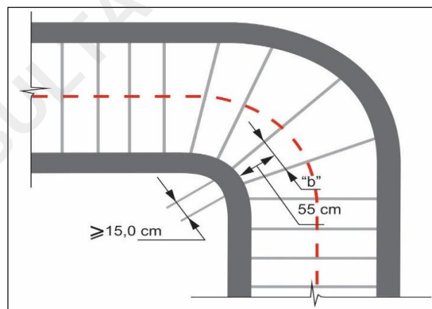
Figura 6: Escada com patamar em leque, degraus balanceados, permitida para acesso a mezaninos e áreas restritas.
