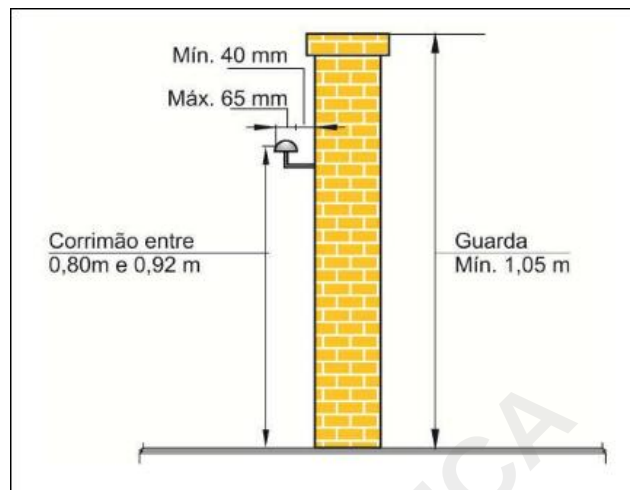
Figura 22: Dimensões de guardas e corrimãos
