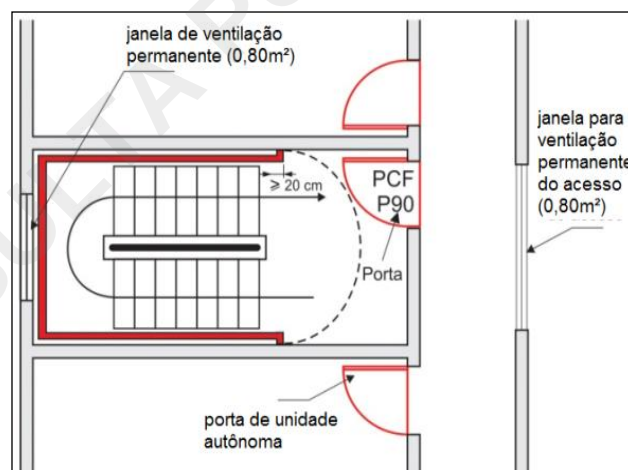
Figura 15: Ventilação da escada enclausurada protegida e seu acesso
