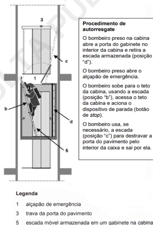
Figura 25: Desenho esquemático do alçapão
