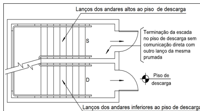
Figura 3: Segmentação das escadas no piso da descarga
