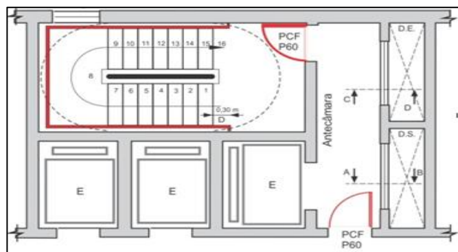
Figura 17: Escada enclausurada à prova de fumaça (demonstração dos dutos)
