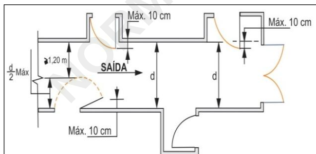
Figura 2: Abertura das portas no sentido de saída
