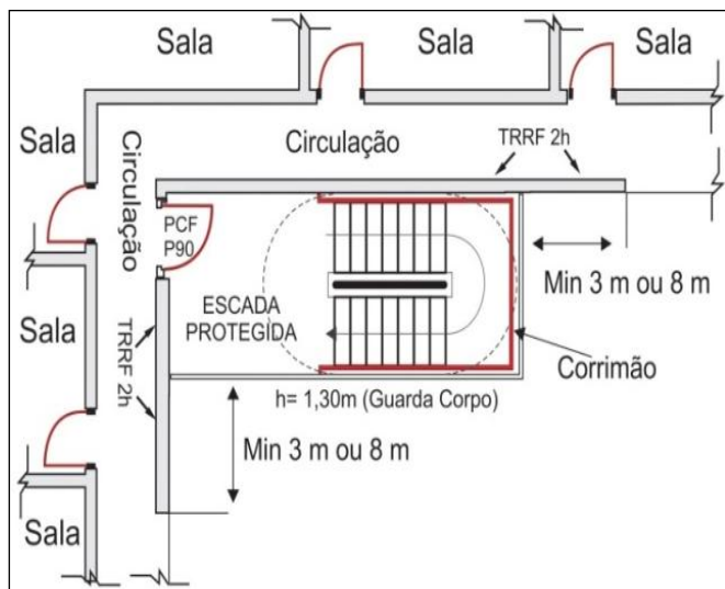
Figura 21: Escada aberta externa
