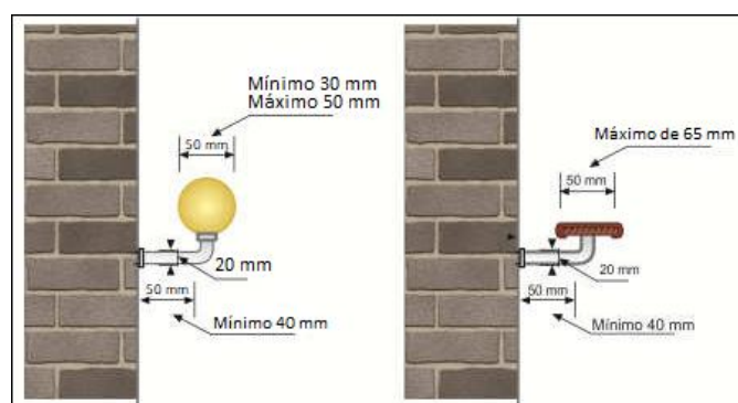
Figura 23: Pormenores de corrimãos
