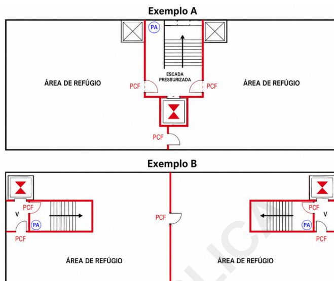
Figura 29: Exemplo esquemático da área de refúgio
