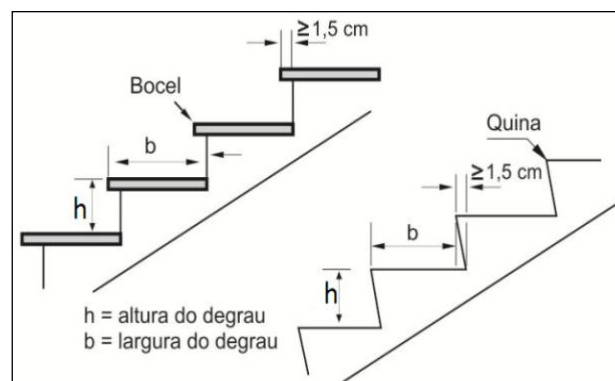
Figura 4: Altura e largura dos degraus
