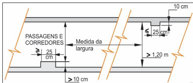
Figura 1: Medida da largura em corredores e passagens
