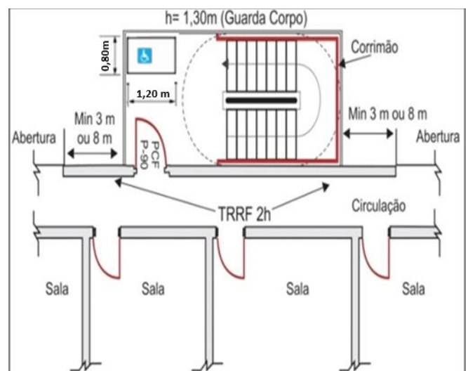
Figura 20: Escada aberta externa
