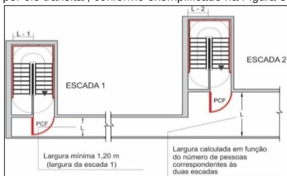
Figura 30: Dimensionamento de corredores de descarga
