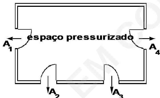
Figura 1: Trajetórias de escape do ar em paralelo
