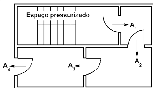
Figura 2: Trajetórias de escape do ar em série
