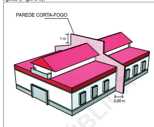
Figura 8: Parede corta-fogo
