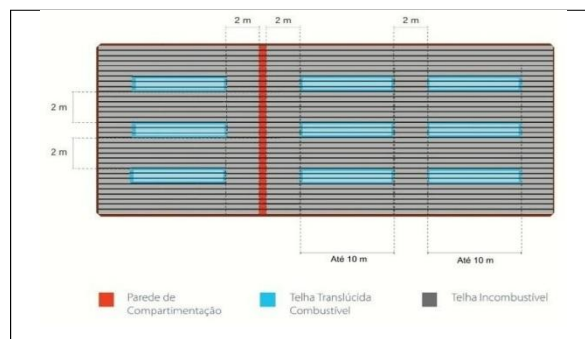
Figura 2: Afastamento de telhas combustíveis translúcidas
