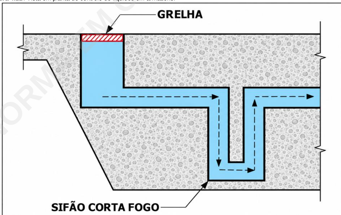
Figura 4.1C: Detalhes do projeto de drenagem de canaletas.
