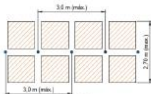
Planta baixa
