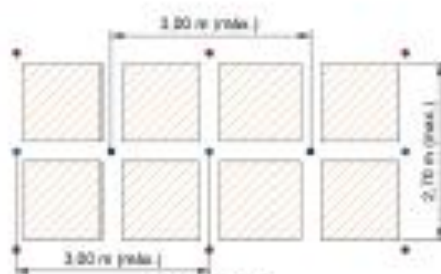
Planta baixa
