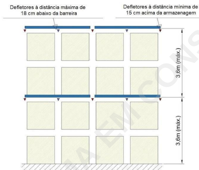
Elevação
